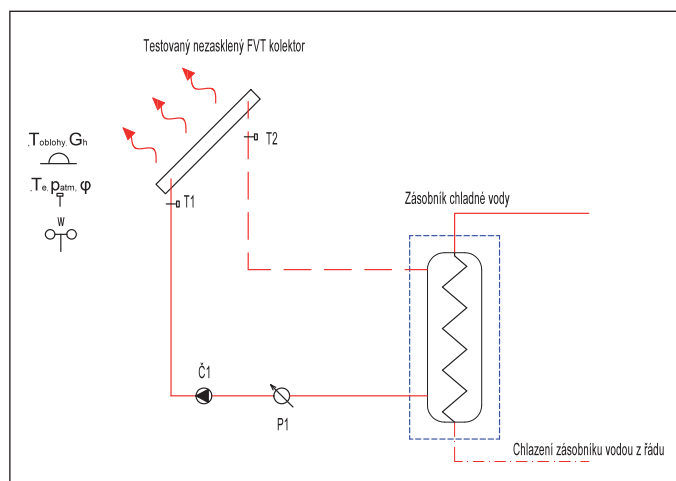
Obr. 4 Schéma zapojení měřicí tratě
