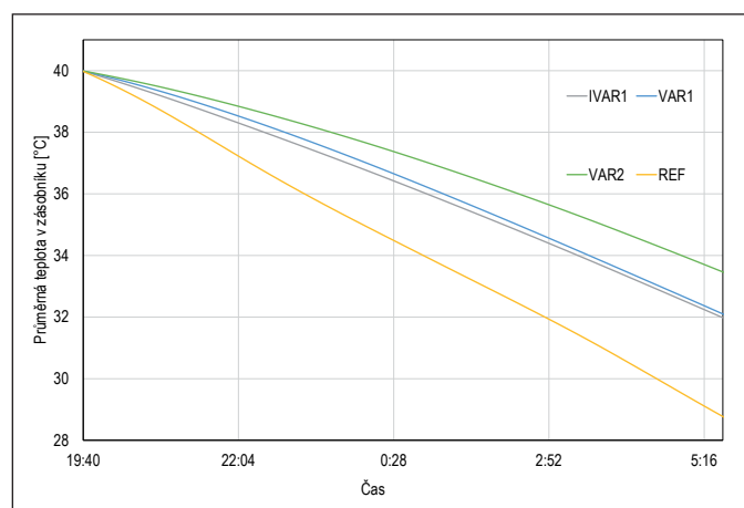
Obr. 9 Noční vychlazování zásobníku (Rijád)
