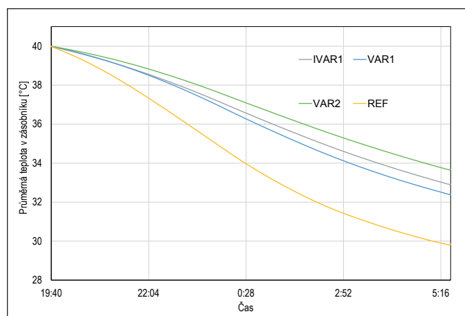
Obr. 10 Noční vychlazování zásobníku (Dubaj)
